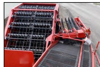
Комбайн SE-260. Сепарирующие элеваторы
